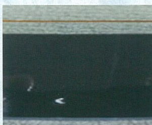
トングマーク例 (ガラス製造掴み跡) (2 mm前後)
